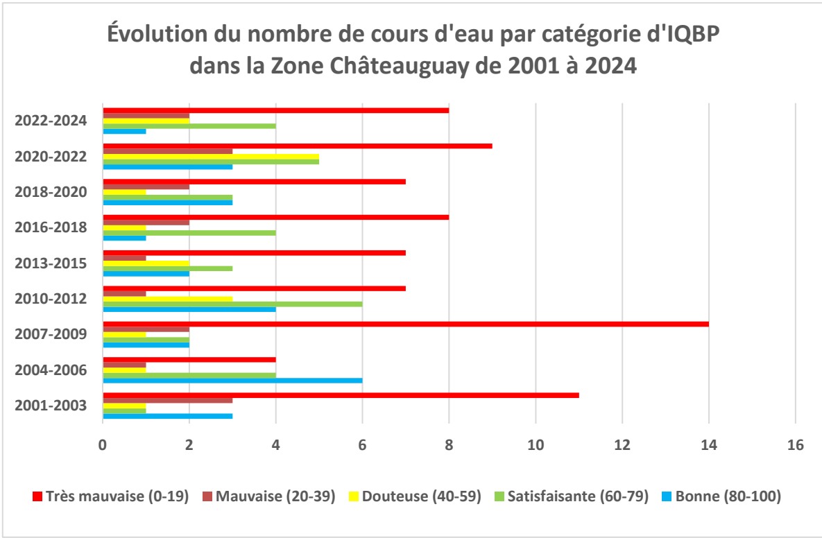
Figure 9 : Qualité de l’eau de surface (IQBP) dans la Zone Châteauguay de 2001 à 2024 42 (MDDELCC, atlas de l’eau 2023 5 )
